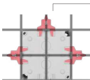
Sistema per il fissaggio alla passerella portacavi. Art. SOP-716Y
