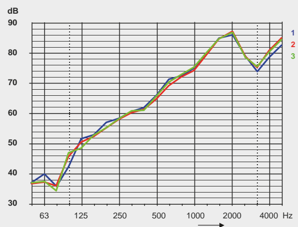
Comparación de los niveles del aislamiento acústico Pared ligera (de 2 capas, cada una con 3 capas de enlucido)
